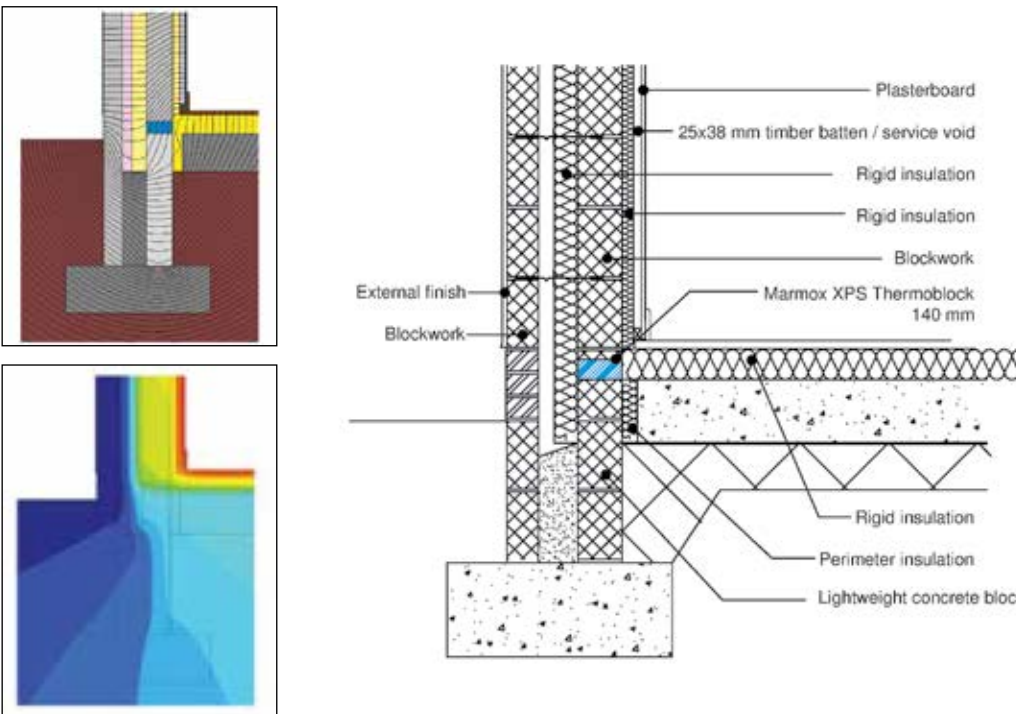
BRE detail 600024
