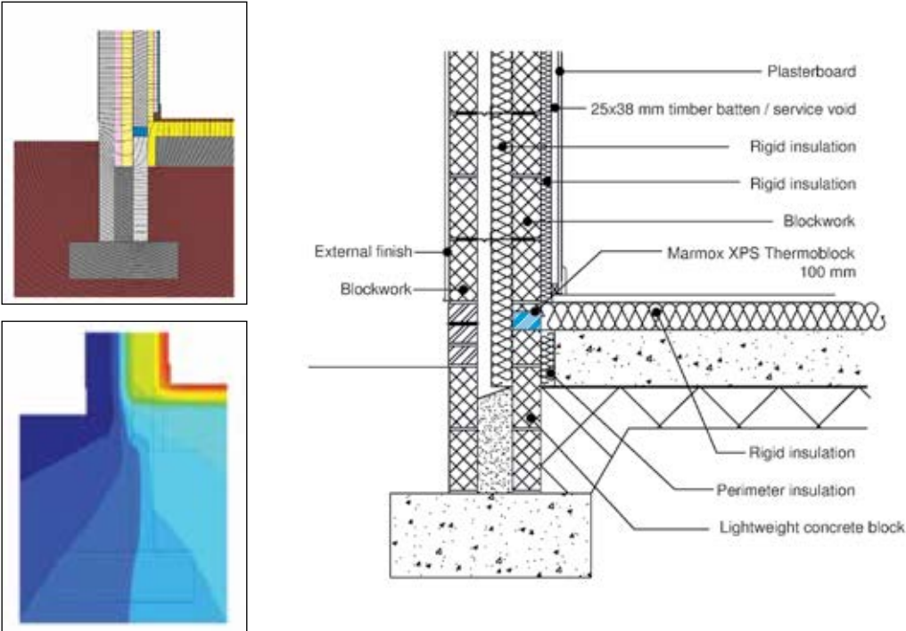
BRE detail 600023
